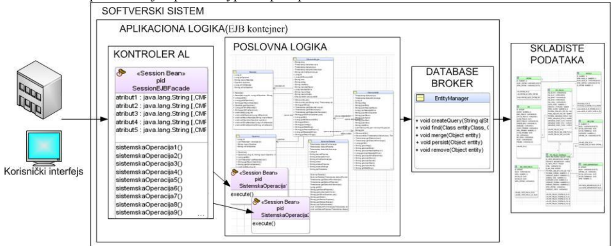
СЛИКА 7 –АРХИТЕКТУРА СОФТВЕРСКОГ СИСТЕМА - СКЛАДИШТЕ ПОДАТАКА
