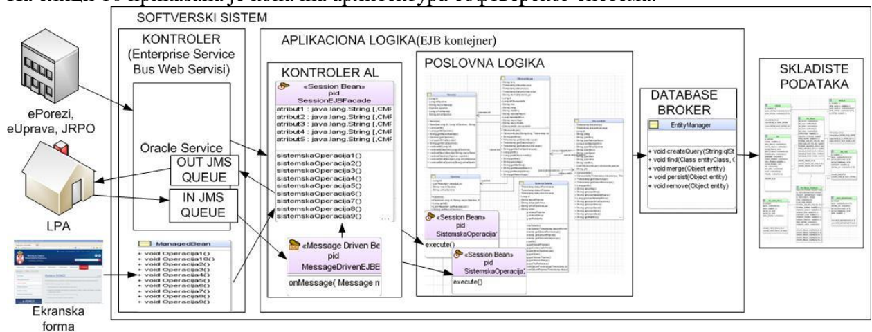
СЛИКА 10 –АРХИТЕКТУРА СОФТВЕРСКОГ СИСТЕМА - КОНАЧАН ИЗГЛЕД
