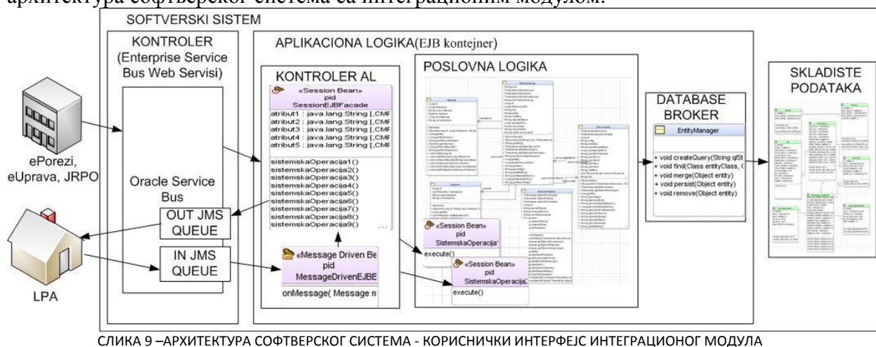
СЛИКА 9 –АРХИТЕКТУРА СОФТВЕРСКОГ СИСТЕМА - КОРИСНИЧКИ ИНТЕГРАЦИОНОГ МОДУЛА
